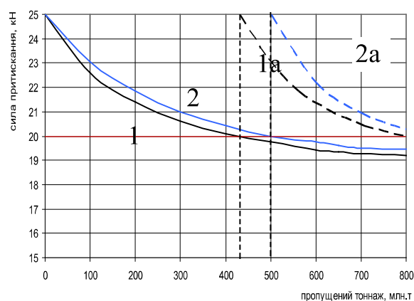
Рис. 2. Графік зміни сили притиснення рейки до шпали у вузлі скріплення КПП-5: 1 – вантажнапруженість 45 млн. т.км/км.рік; 2 – вантажнапруженість 60 млн. т.км/км.рік; 1a, 2a – зміна сили притиснення після укладання нових прокладок
