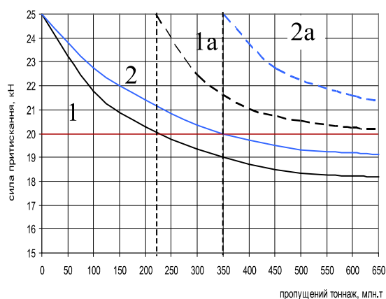
Рис. 1. Графік зміни сили притиснення рейки до шпали у вузлі скріплення КПП-5: 1 – вантажнапруженість 15 млн. т.км/км.рік; 2 – вантажнапруженість 30 млн. т.км/км.рік; 1a, 2a – зміна сили притиснення після укладання нових прокладок
