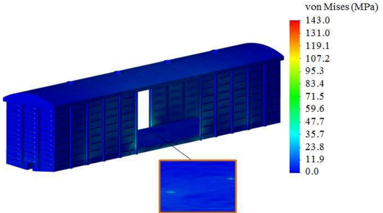
Рис. 4. Напружений стан кузова критого вагона
