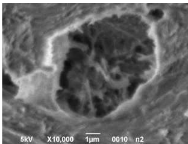
Рис. 4. Электронно-микроскопические снимки сколов портландцементного камня: а – без добавок; б – с ХАД и НМОС (округлая область размером 5–7 мкм – отверстие, из которого при раскалывании «вырвано» волокно)
