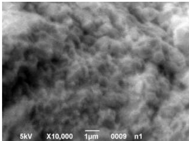
Рис. 4. Электронно-микроскопические снимки сколов портландцементного камня: а – без добавок; б – с ХАД и НМОС (округлая область размером 5–7 мкм – отверстие, из которого при раскалывании «вырвано» волокно)
