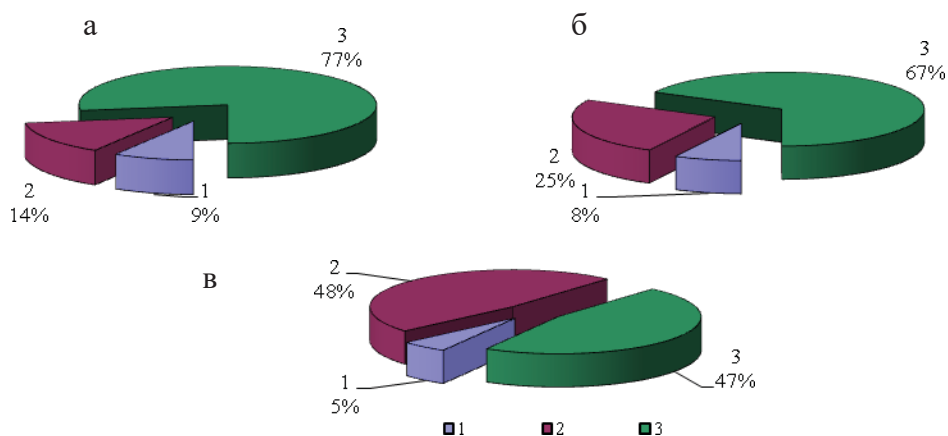
Рис. 1. Співвідношення формуючих сумарну поздовжню силу угону при конструкції колії з рейковими скріпленнями КПП-5 та епюрою укладання шпал 1840 шт/км: а – при службовому гальмуванні; б – при екстремому гальмуванні; в – при рекуперативному гальмуванні; 1 – сила від пружного вигину рейки; 2 – гальмівна сила; 3 – температурна сила.
