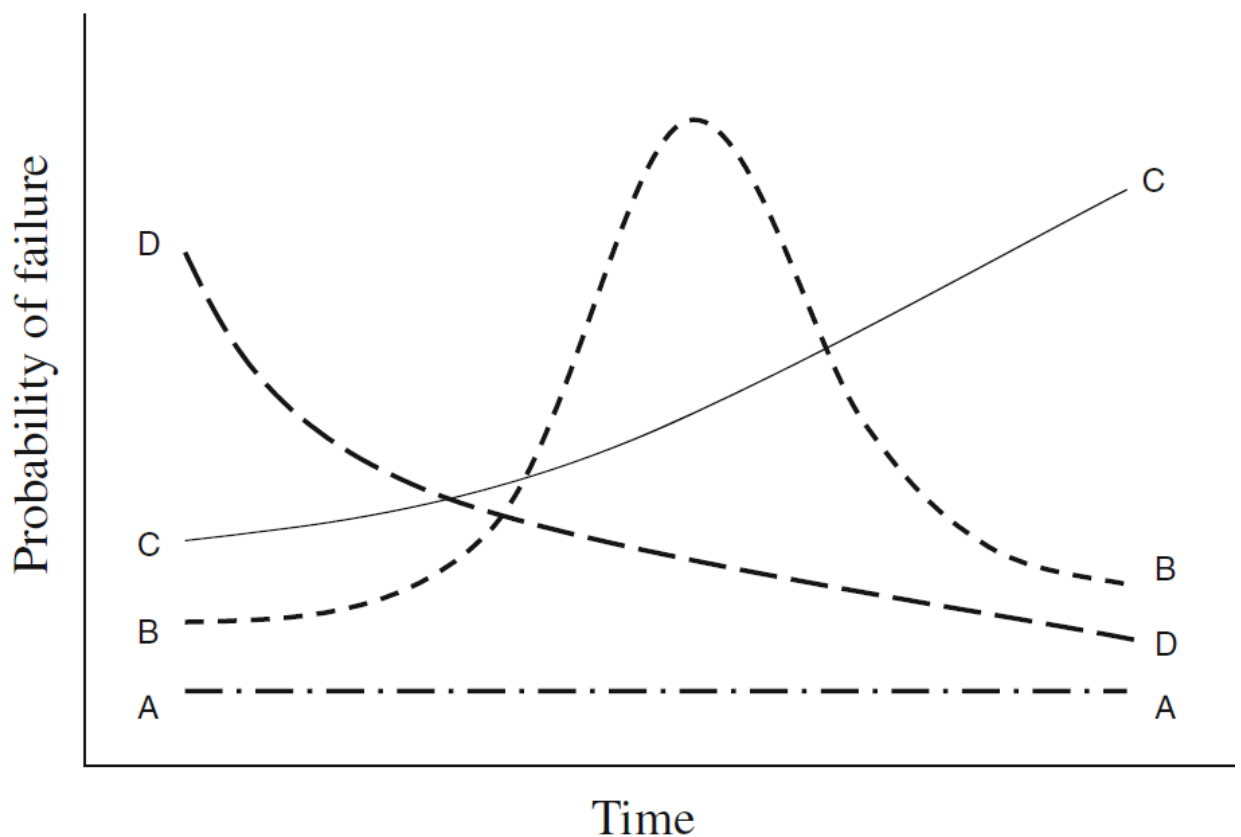
Рисунок 1.3 – Типові криві розподілу ймовірності відмов вузлів у часі
