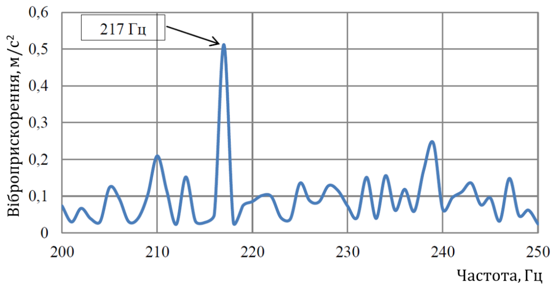
Рисунок 4.5 – Спектр обвідної вібрації із ознаками пошкодження внутрішнього кільця підшипника
