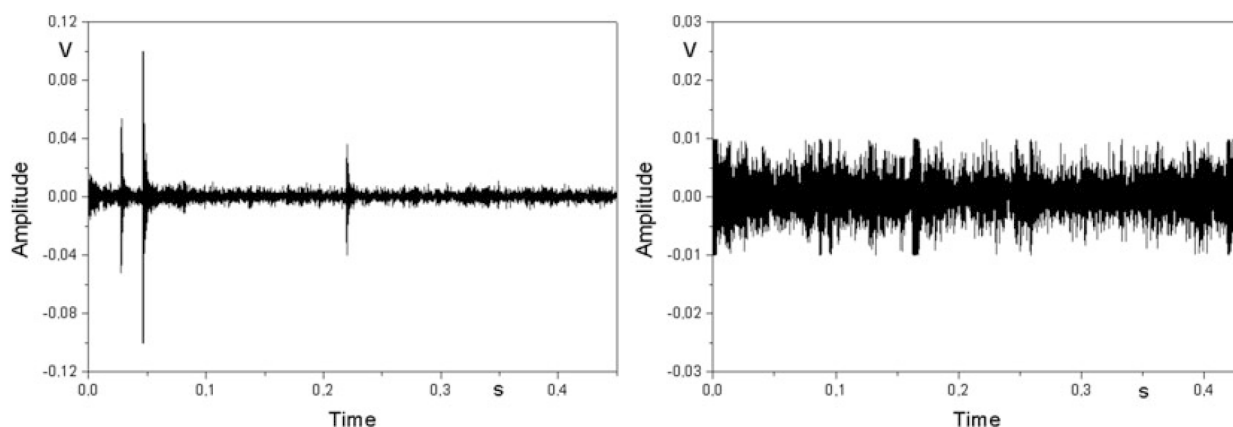
Рисунок 3.6 – Часові реалізації сигналів перехідної імпульсної акустичної емісії та безперервної акустичної емісії [2]
