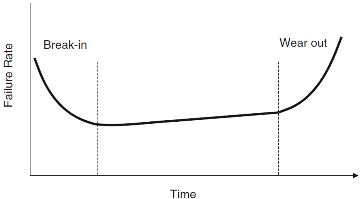
Рисунок 1.2 – Трифазна крива зміни інтенсивності відмов у часі.
