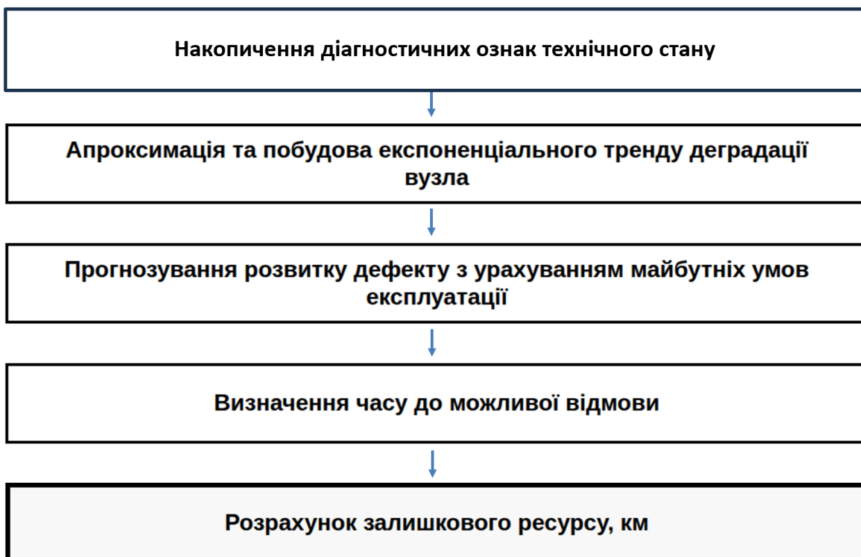
Рисунок 4.9 – Послідовність визначення деградації підшипникового вузла
