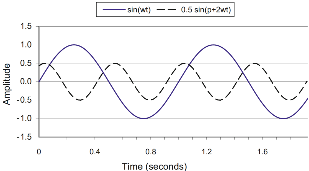
Рисунок 3.2 – Хвилі синусоїд
